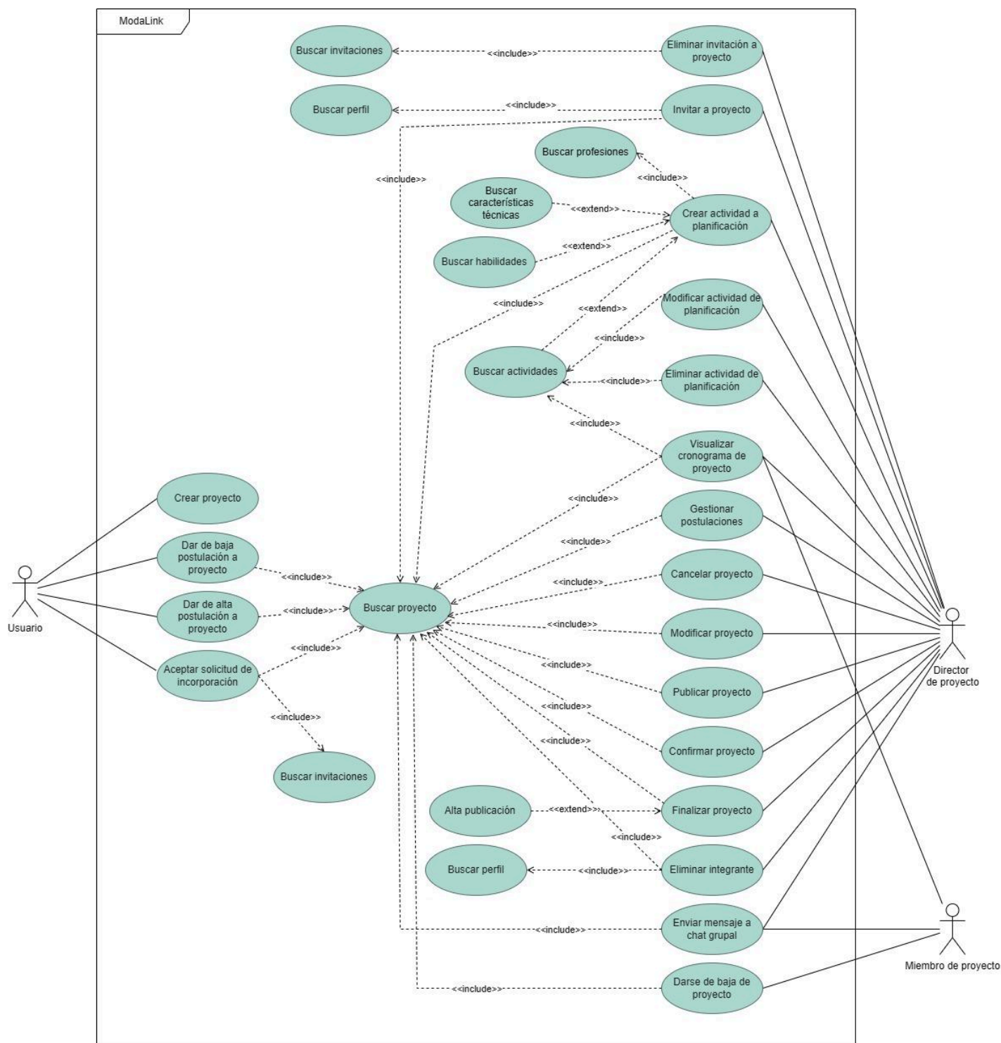
Figura 5 - Diagrama de Casos de Uso - “Gestión de proyectos”
