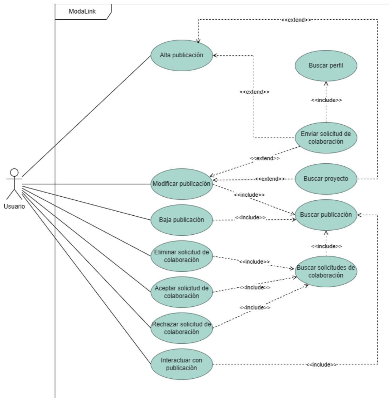
Figura 11 - Diagrama de Casos de Uso - “Gestión de publicaciones”
