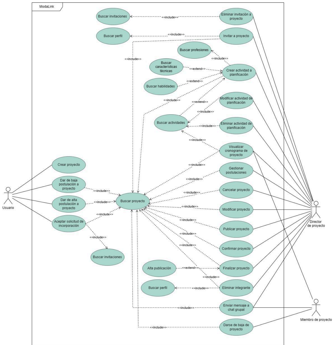
Figura 12 - Diagrama de Casos de Uso - "Gestión de proyectos"
