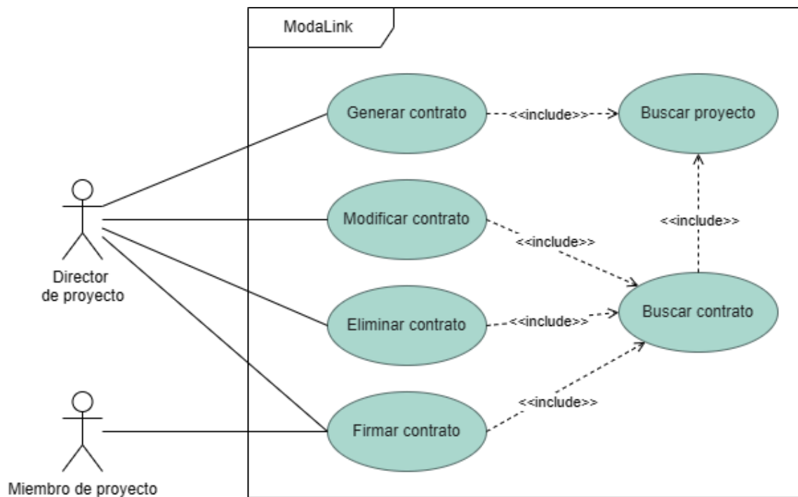
Figura 13 - Diagrama de Casos de Uso - “Gestión de contratos”
