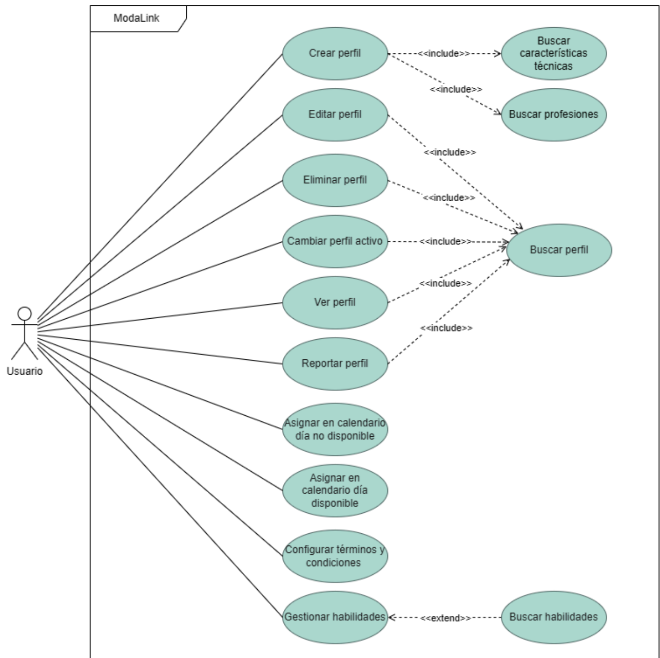
Figura 10 - Diagrama de Casos de Uso - “Gestión de perfiles”
