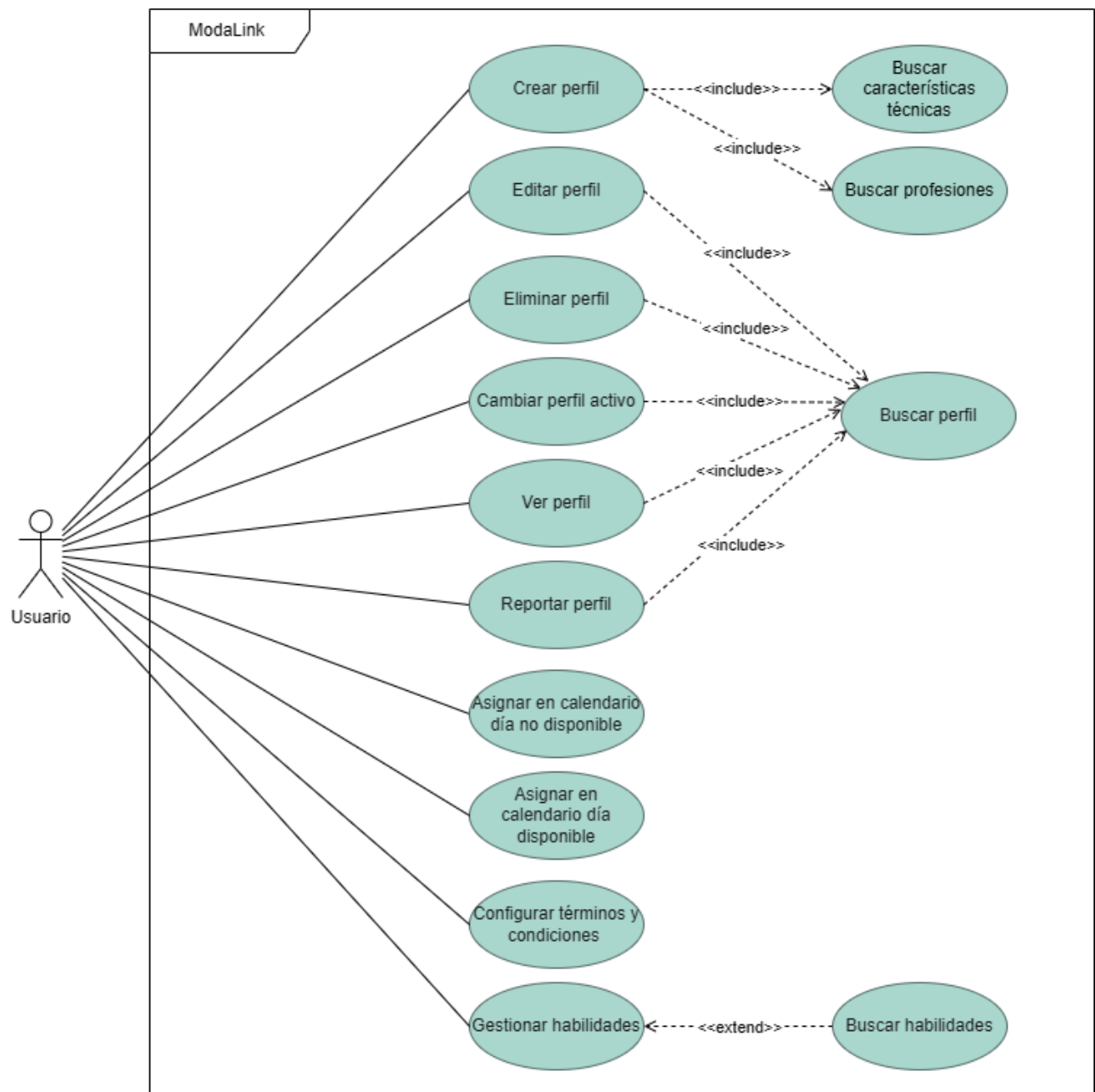
Figura 3 - Diagrama de Casos de Uso - “Gestión de perfiles”
