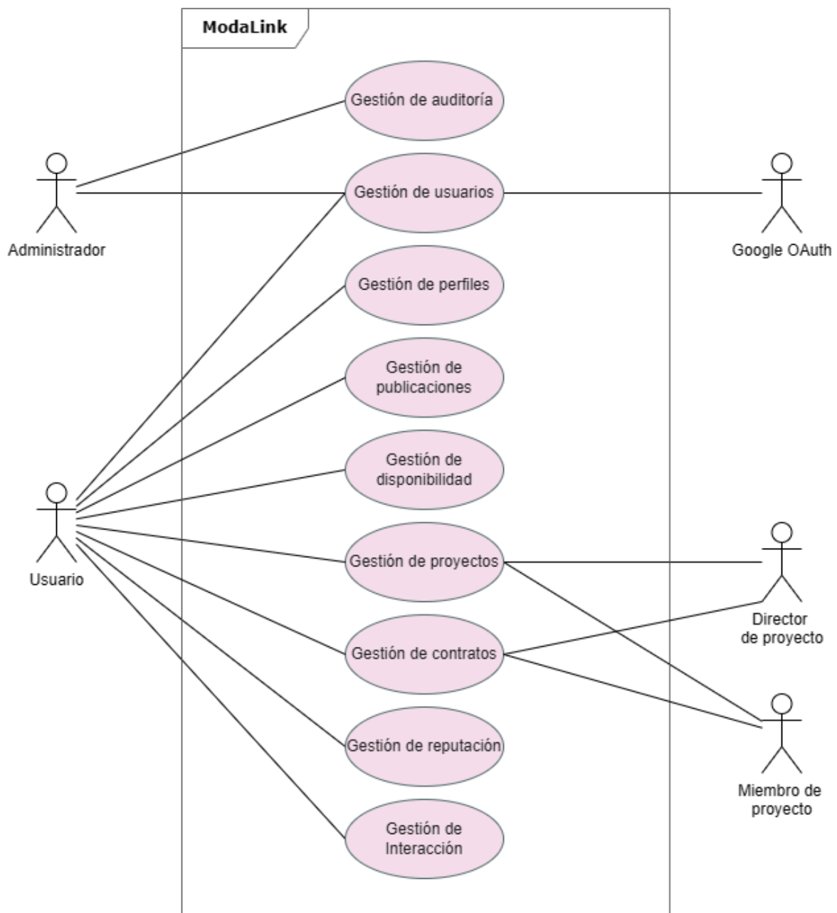
Figura 1- Diagrama de Casos de Uso de alto nivel - Diagrama de contexto
