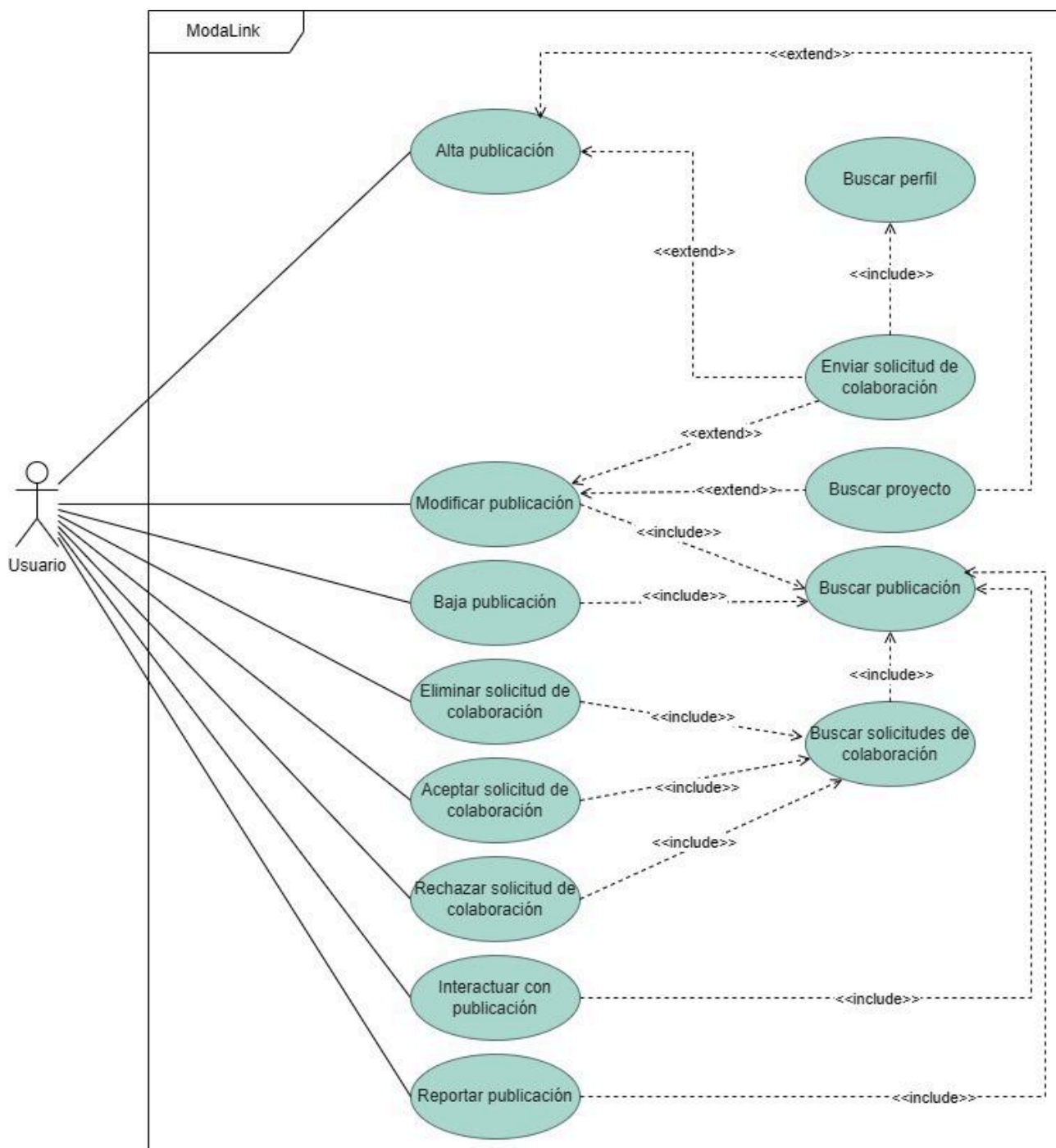
Figura 4 - Diagrama de Casos de Uso - “Gestión de publicaciones”
