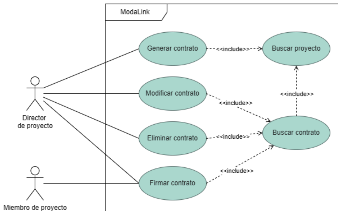
Figura 6 - Diagrama de Casos de Uso - “Gestión de contratos”
