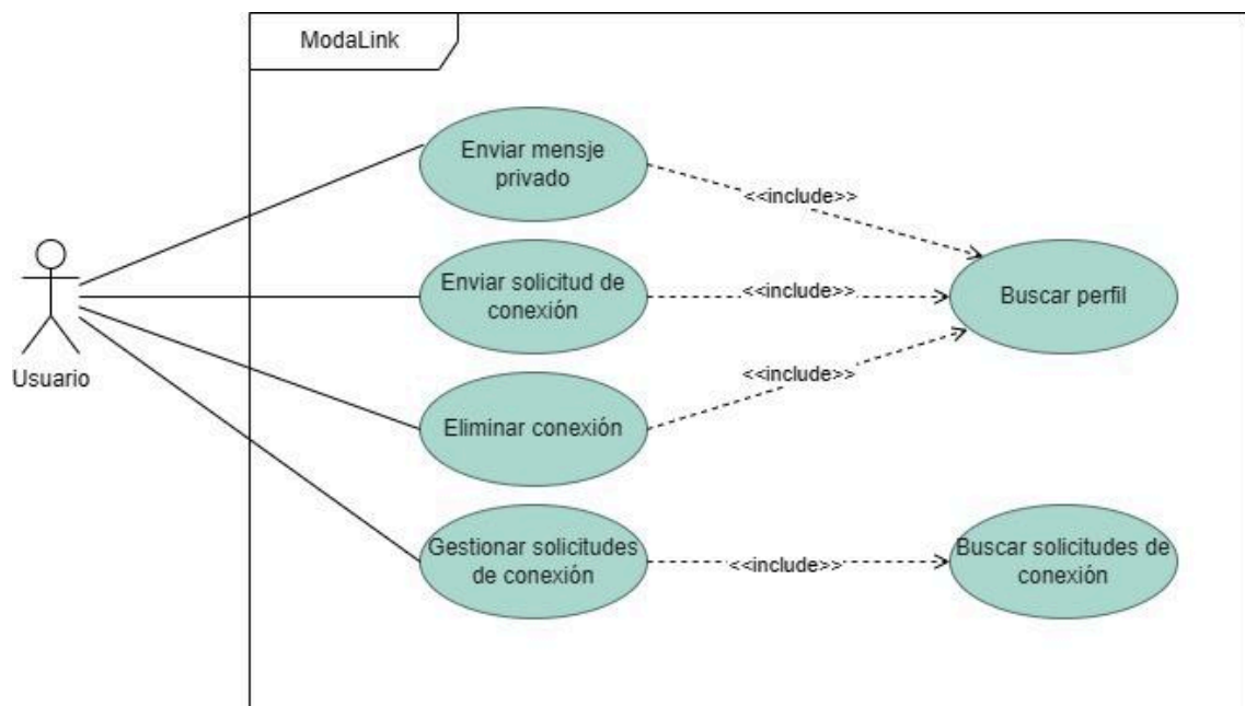
Figura 14 - Diagrama de Casos de Uso - “Gestión de conexiones y mensajería”
