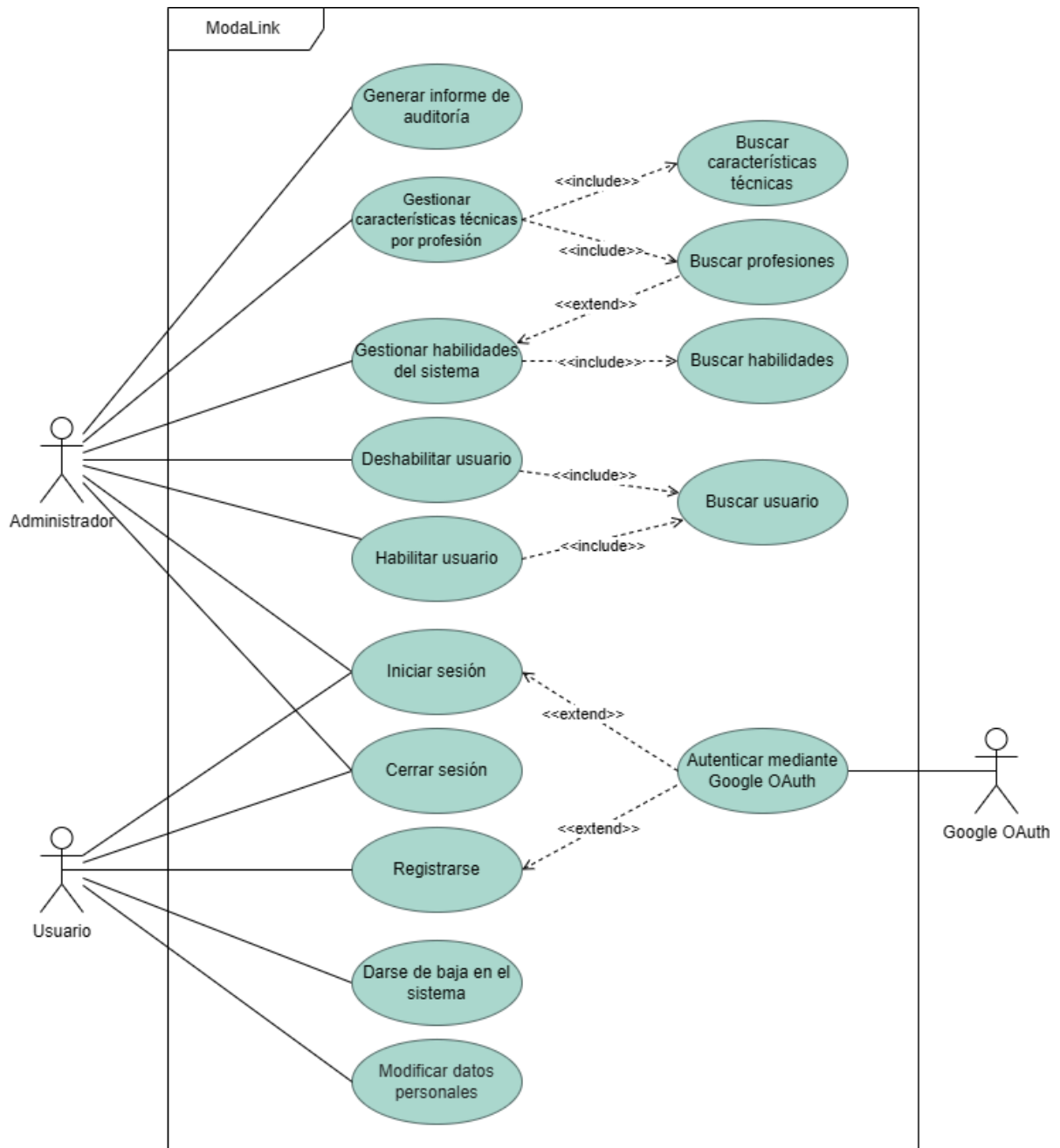
Figura 9 - Diagrama de Casos de Uso - “Gestión de usuarios”
