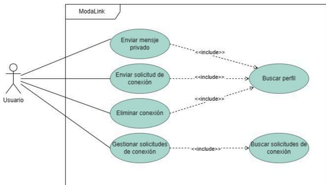
Figura 7 - Diagrama de Casos de Uso - “Gestión de conexiones y mensajería”
